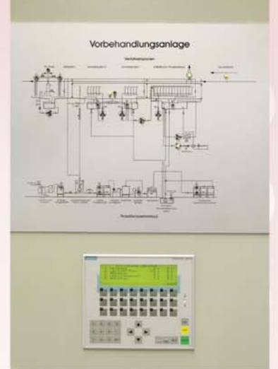
Steuerzentrale Vorbehandlung
